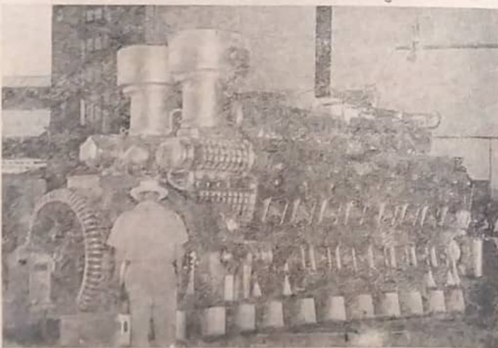
Novo motor gerador Diesel de 1.000 KW. que a partir de 15 de março de 1952 entrou em serviço, aumentando a capacidade da usina geradora da THE RIO GRANDENSE LIGHT & POWER SYNDICATE, LIMITED
